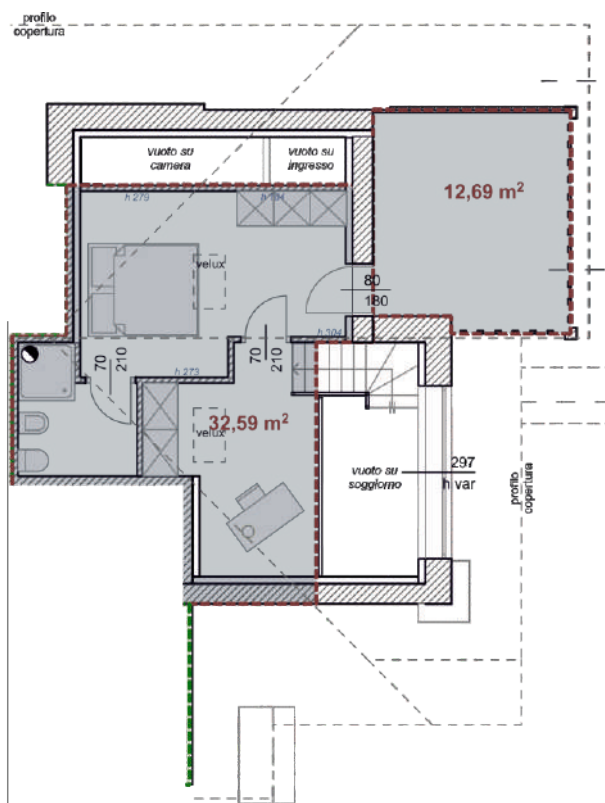
PIANO SECONDO SOTTOTETTO
