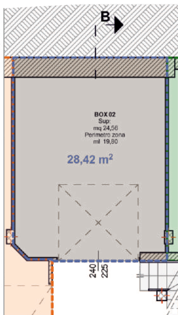
PIANO PRIMO INTERRATO
