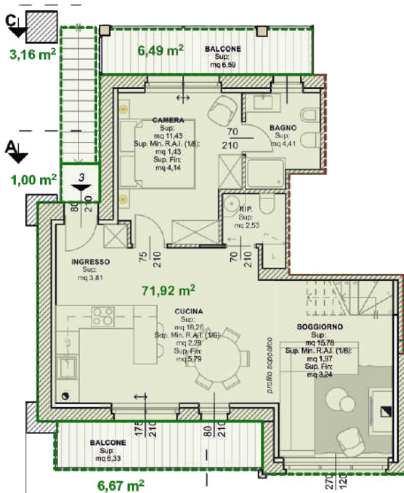
PIANO PRIMO
