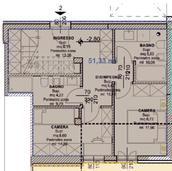
PIANO PRIMO INTERRATO
