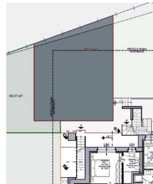
PIANIMETRIA
